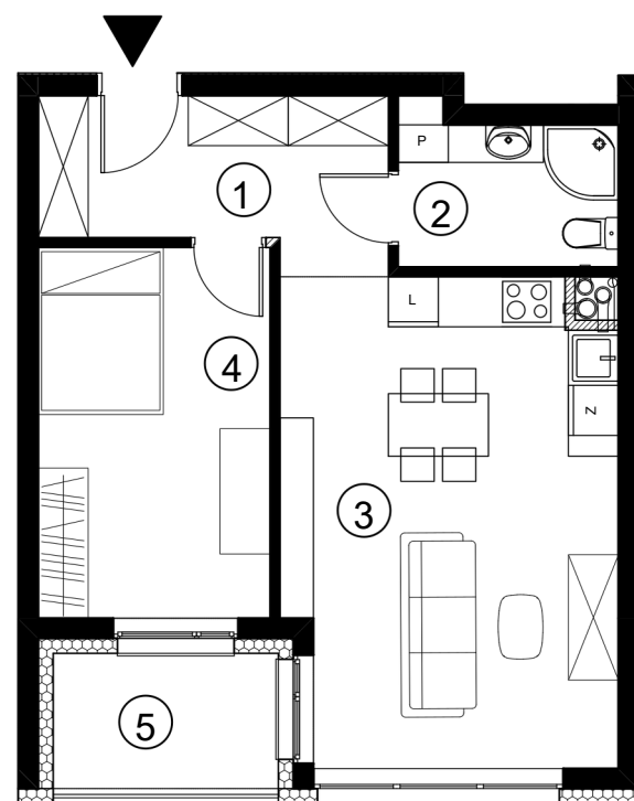
II piętro
