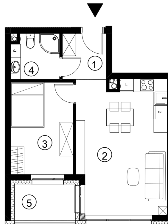
II piętro
